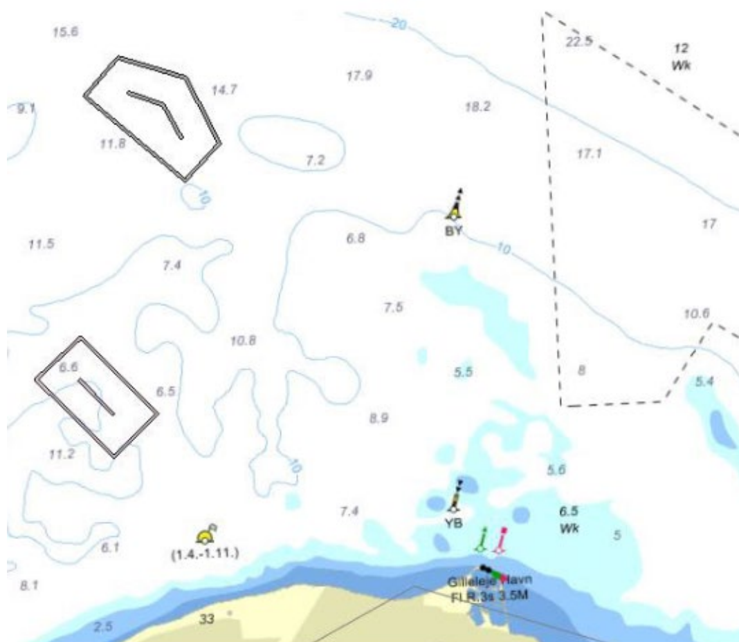
Figur 10.2: Projektområdet for Statens etablering af nye stenrev er inddelt i 2 områder på Gilleleje Flak nordvest for Gilleleje.
